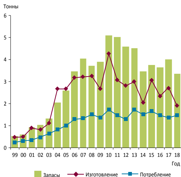
Рис. XI. Фентанил: мировое изготовление, потребление и запасы a , 1999–2018 годы
